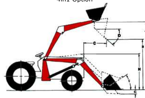
4in1 Option
